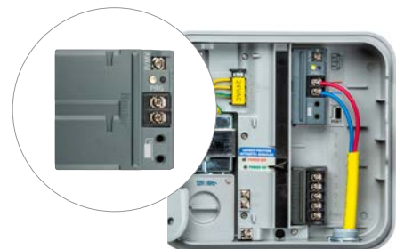
Pro-C Decoder-Ausgangsmodul
